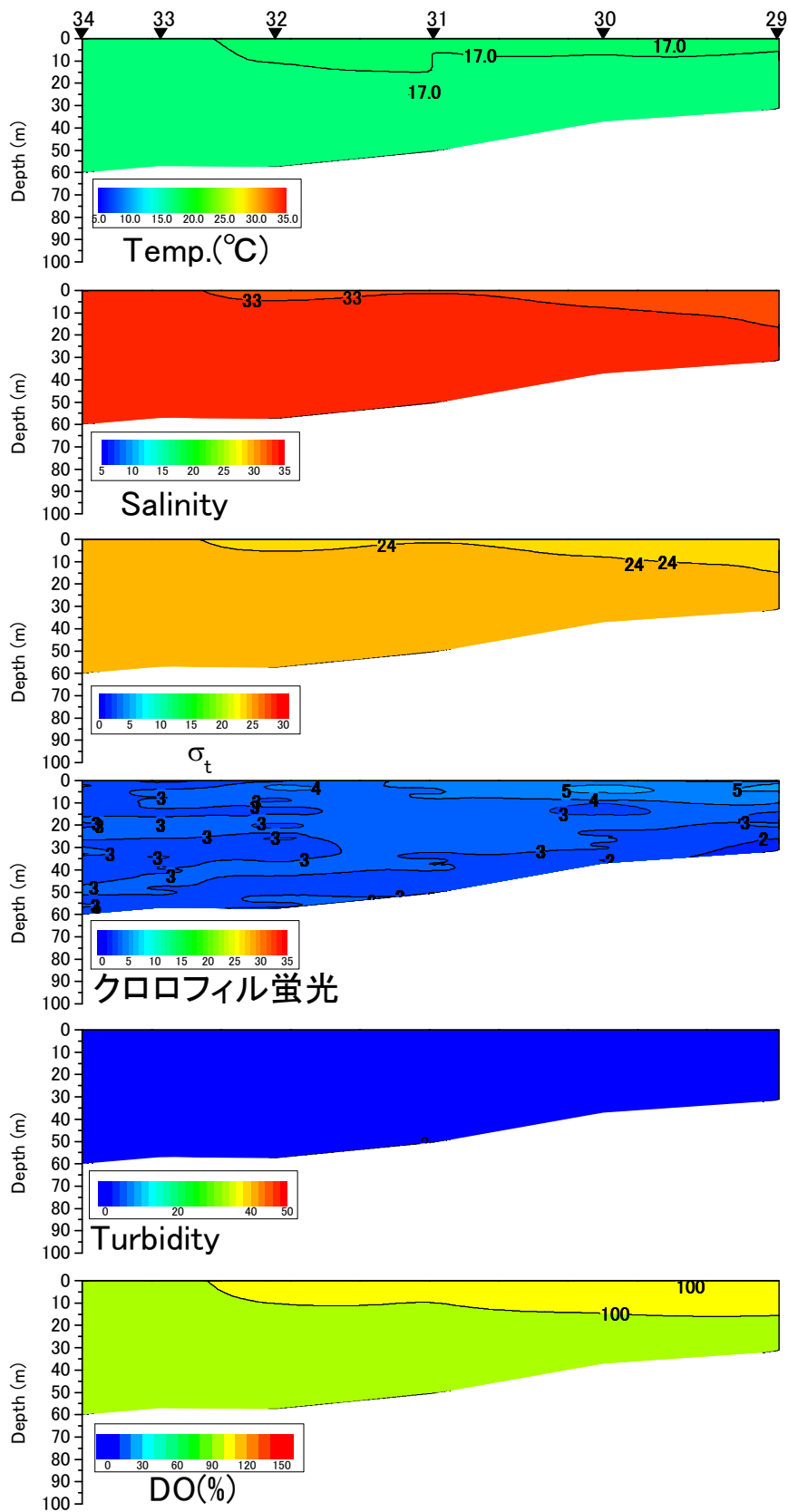
八代海西ラインの水温(°C)、塩分、密度( \sigma_t )、クロロフィル蛍光強度、濁度、溶存酸素飽和度(DO%)の鉛直面図(国土交通省の調査による) (2017年4月26日)
